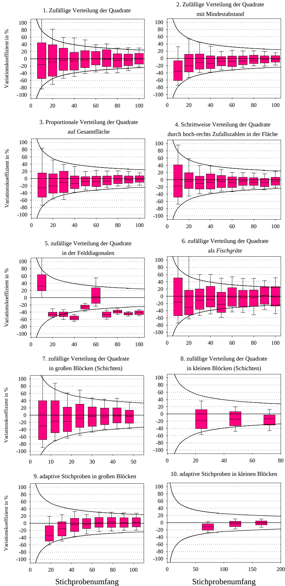
Anlage C: Beobachtete Streuung des Populationsschätzers aus 200 Wiederholungen im Vergleich zur erwarteten Streuung für die Natternzunge, Seidenbachtal
