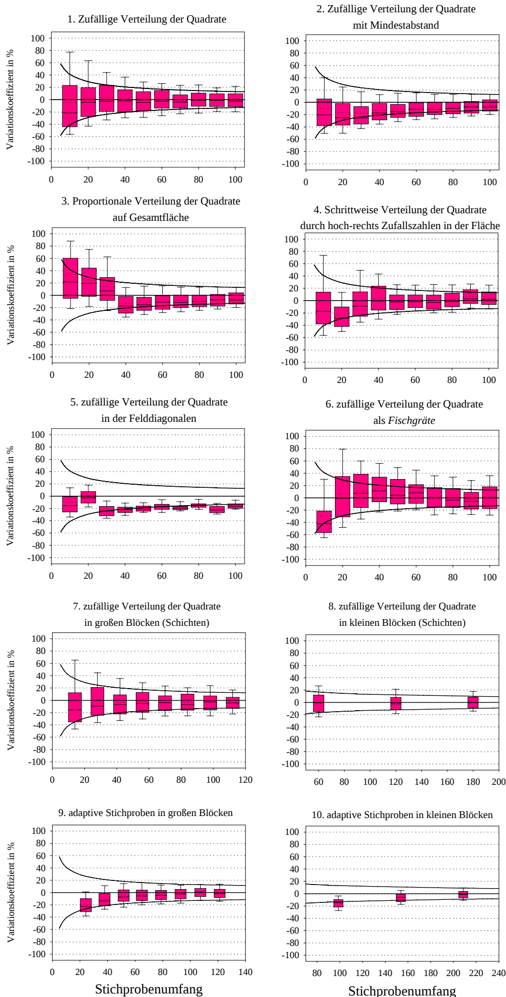
Anlage C: Beobachtete Streuung des Populationsschätzers aus 200 Wiederholungen im Vergleich zur erwarteten Streuung für die Gelbe Narzisse, M2
